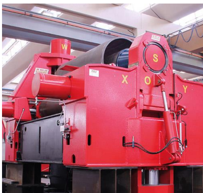
Krivilni stroj na 3 valje – MAV 3000 mm x 136 mm
